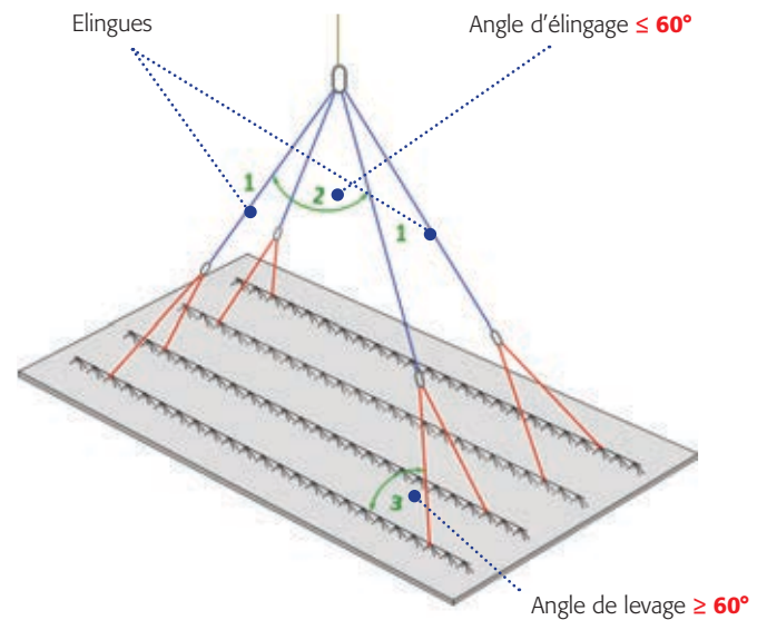
■ Inclinaison des élingues : angle d'élingage et de levage
