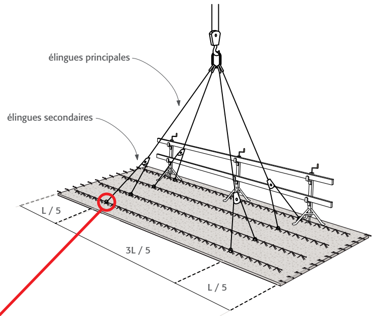
■ Dispositif de manutention : position des crochets de levage
