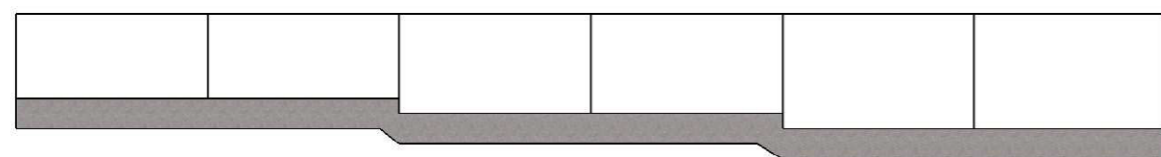
MUR HORIZONTAL SUR SEMELLE EN REDANT
