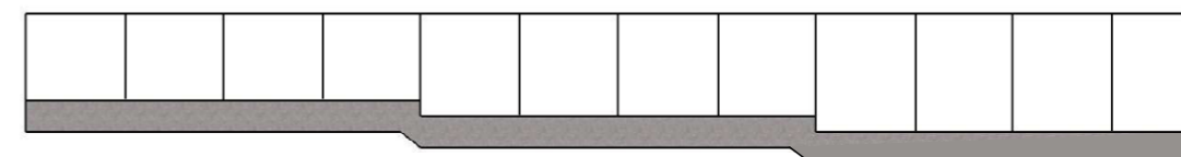
MUR HORIZONTAL SUR SEMELLE EN REDANT
